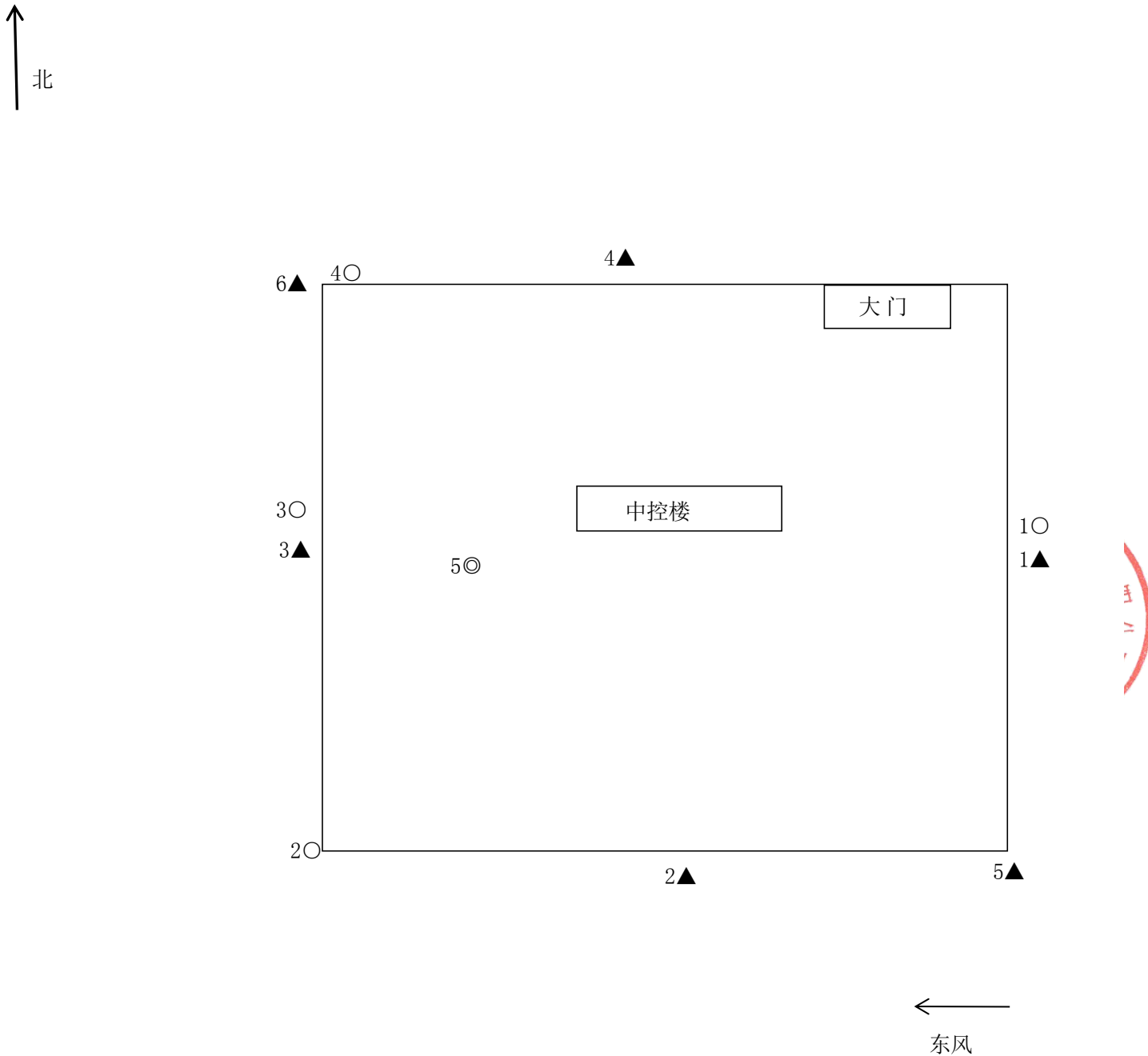
附图:检测点位图
